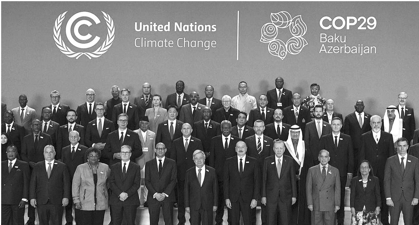
● COP29 đánh dấu một cột mốc quan trọng với việc thông qua khuôn khổ thị trường carbon toàn cầu. (Ảnh: UNFCCC)
