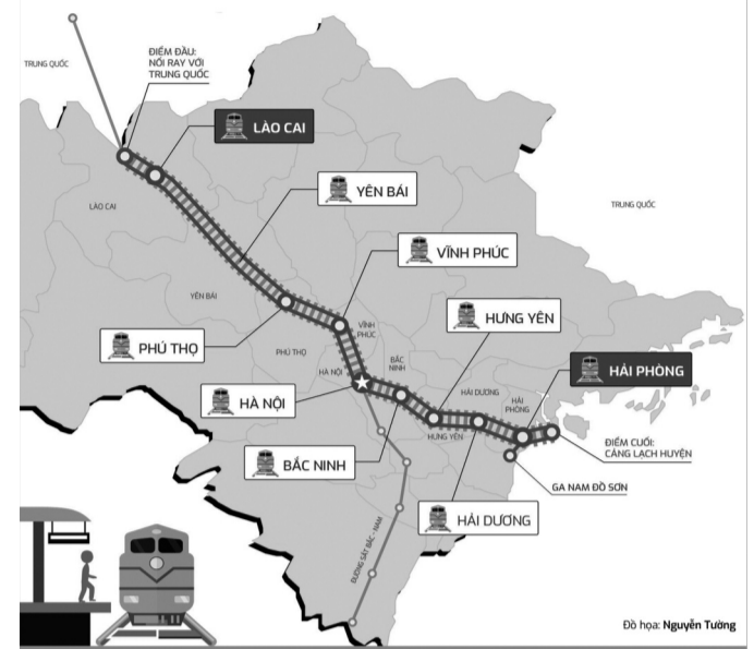
● Hướng tuyến đường sắt Lào Cai - Hà Nội - Hải Phòng khổ 1.435mm theo Báo cáo nghiên cứu tiền khả thi.
