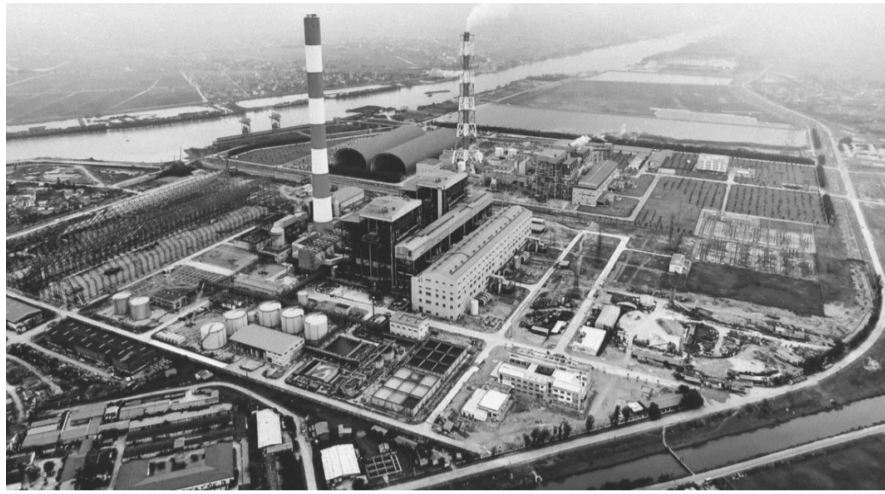
● Nhà máy Nhiệt điện Thái Bình 2 cán mốc sản lượng 10 tỷ kWh. (Ảnh: Petrovietnam)
